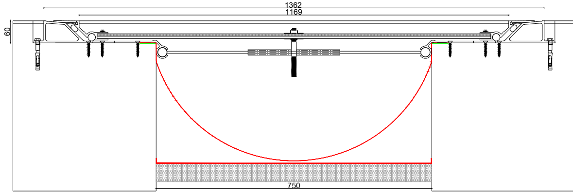
■ Z-5000 W-750W1362 JW : 750 H: 60 S: 1362 BW: 1420 M: 1001
