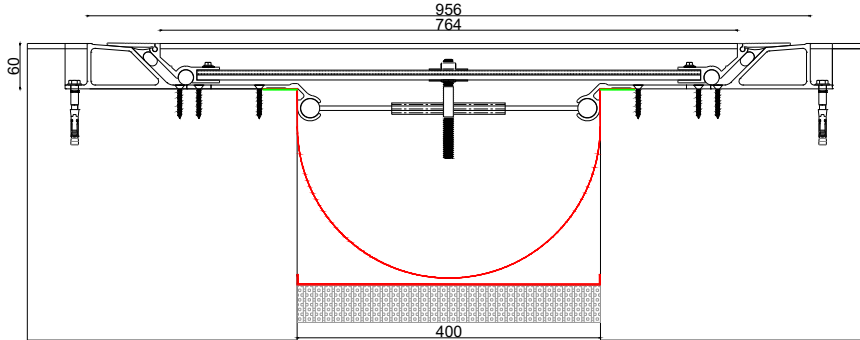
■ Z-5000 W-400W956 JW : 400 H: 60 S: 956 BW: 1014 M: 668
