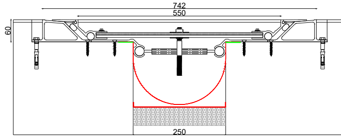
■ Z-5000 W-250W742 JW : 250 H: 60 S: 742 BW: 800 M: 450
