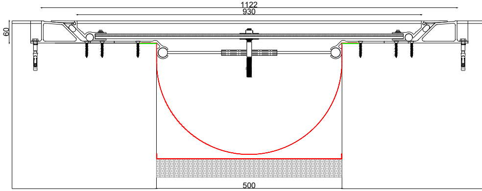
■ Z-5000 W-500W1122 JW : 500 H: 60 S: 1122 BW: 1180 M: 832
