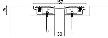
■ Z-6000-30W157 JW : 30 H: 25 S: 157 M: 60
