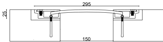
■ Z-6000-150W295 JW : 150 H: 25 S: 295 M: 80
