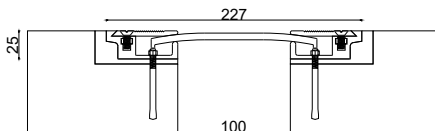
■ Z-6000-100W227 JW : 100 H: 25 S: 227 M: 60
