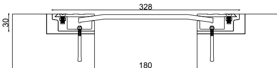
■ Z-6000-180W328 JW : 180 H: 30 S: 328 M: 80
