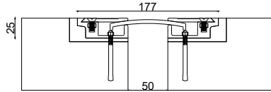
■ Z-6000-50W177 JW : 50 H: 25 S: 177 M: 60
