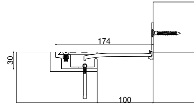
■ ZK-6000-100W174 JW : 100 H: 30 S: 174 M: 40
