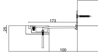
■ ZK-6000-100W173 JW : 100 H: 25 S: 173 M: 40
