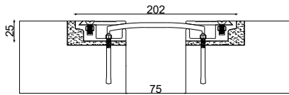
■ Z-6000-75W202 JW : 75 H: 25 S: 202 M: 60
