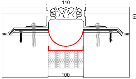
■ Z-1900-100W110 JW : 100 H: 60 S: 110 M: 20
