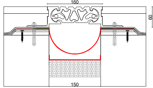
■ Z-1900-150W160 JW : 150 H: 60 S: 160 M: 30
