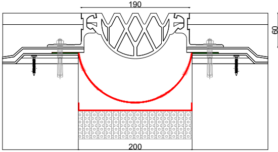
■ Z-1900-200W190 JW : 200 H: 60 S: 190 M: 50
