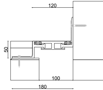
■ ZK-1520-100W120 JW : 100 H: 50 S: 120 BW: 180 M: 15
