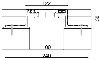
■ Z-1520-100W122 JW : 100 H: 50 S: 122 BW: 240 M: 15
