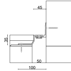
■ ZK-1520-50W45 JW : 50 H: 35 S: 45 BW: 100 M: 8
