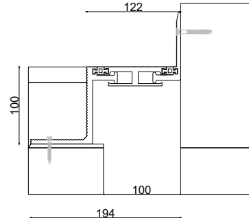
■ ZK-1520-100W122 JW : 100 H: 100 S: 122 BW: 194 M: 15
