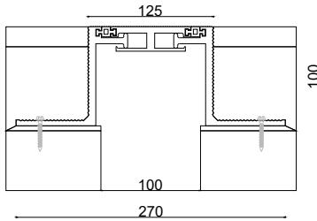
■ Z-1520-100W125 JW : 100 H: 100 S: 125 BW: 270 M: 15
