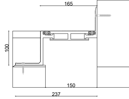
■ ZK-1520-150W165 JW : 150 H: 100 S: 165 BW: 237 M: 8
