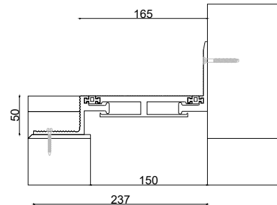
■ ZK-1520-150W165 JW : 150 H: 50 S: 165 BW: 237 M: 15
