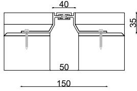
■ Z-1520 -50W40 JW : 50 H: 35 S: 40 BW: 150 M: 8
