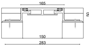
■ Z-1520-150W165 JW : 150 H: 50 S: 165 BW: 283 M: 15
