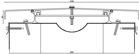
R 2001-200W430 JW :200 H:40 S:430 BW:430 M:200
