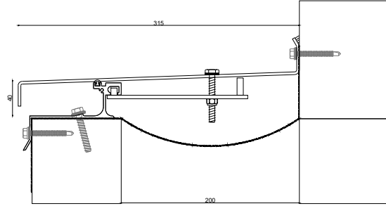
RK 2001-200W315 JW :200 H:40 S:315 BW:315 M:200
