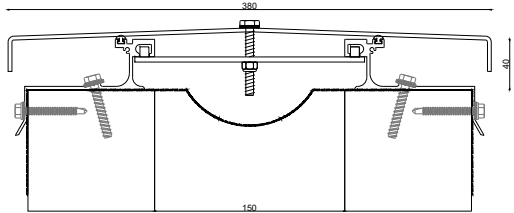
R 2001-150W380 JW :150 H:40 S:380 BW:380 M:150
