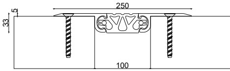
OF-1900-100W250 JW : 100 H: 33 / 5 S: 250 M: 15
