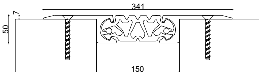
OF-1900-150W341 JW : 150 H: 50 / 7 S: 341 M: 25
