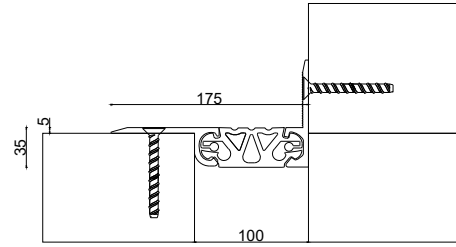
OFK-1900-100W175 JW : 100 H: 35 / 5 S: 175 M: 15
