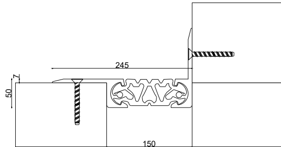
OFK-1900-150W245 JW : 150 H: 50 / 7 S: 245 M: 25
