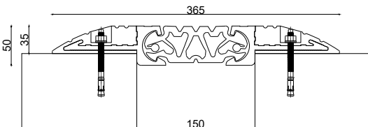
OF-1900-150W365 JW : 150 H: 50 / 35 S: 365 M: 25
