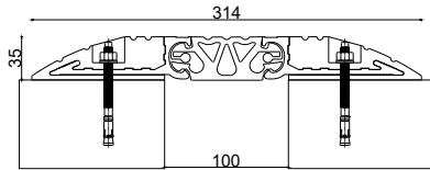
OF-1900-100W314 JW : 100 H: 35 S: 314 M: 15
